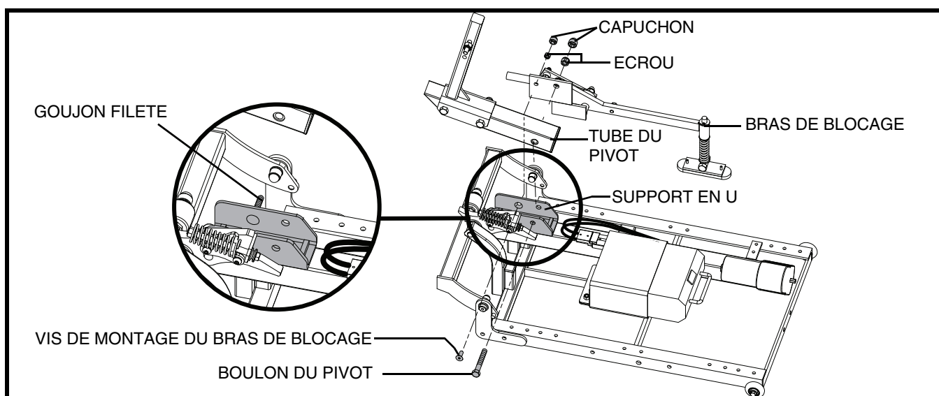
Figure 4. Installation du bras de blocage
