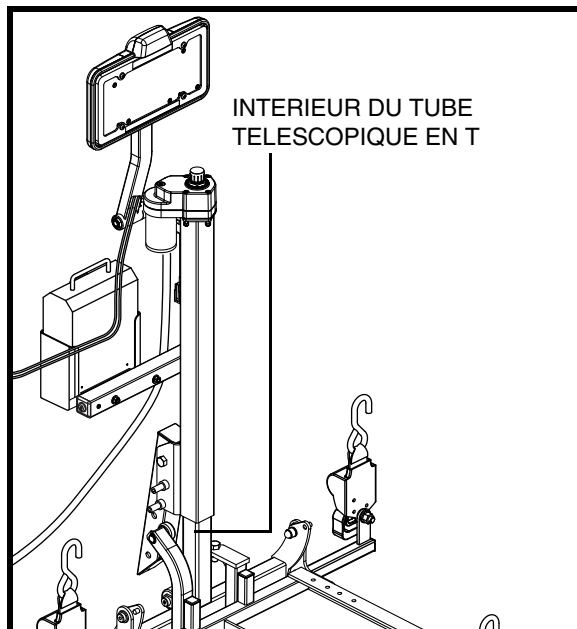
Figure 21. Entretien de la structure de l'appareil de levage
