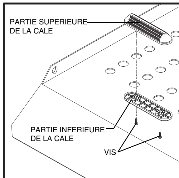
Figure 10. Installation des cales de roues
