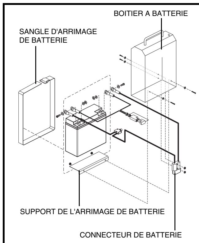
Figure 20. Remplacement d'une batteries
