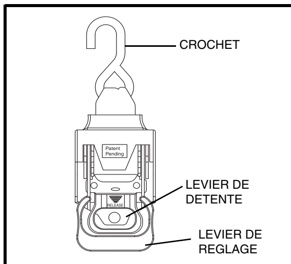
Figure 12. Courroie d'ancrage rétractable
