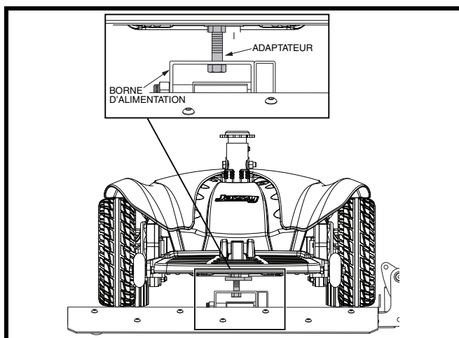
Figure 17. Fauteuil motorisé embarqué
