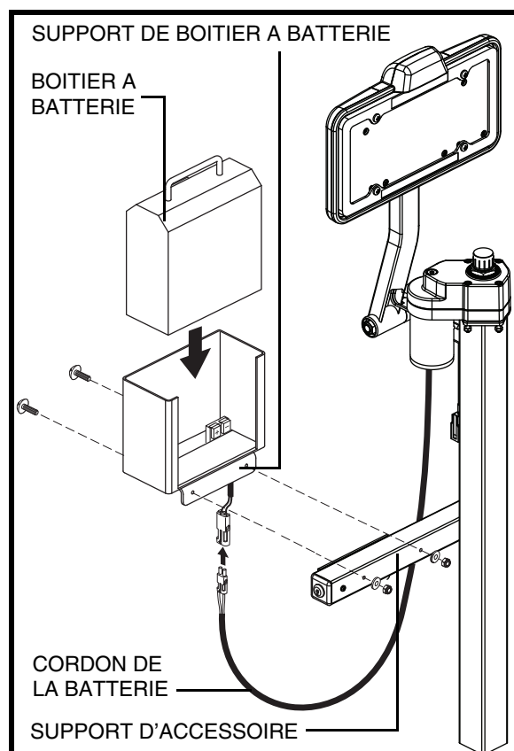
Figure 9. Installation de la batterie interne
