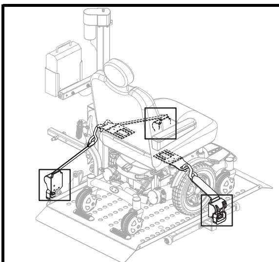
Figure 14. Fixation des courroies d'ancrage rétractable
