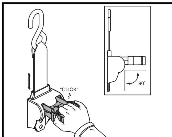
Figure 13. Déverrouillage des courroies d'ancrage rétractable
