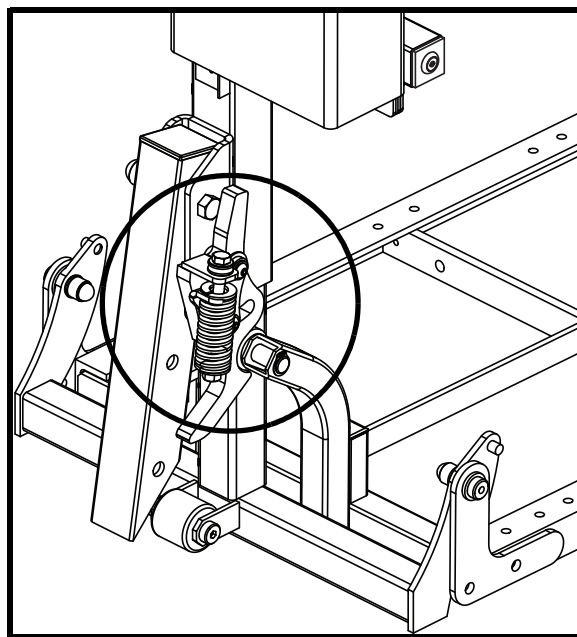
Figure 22. Commutateur mécanique à ressort
