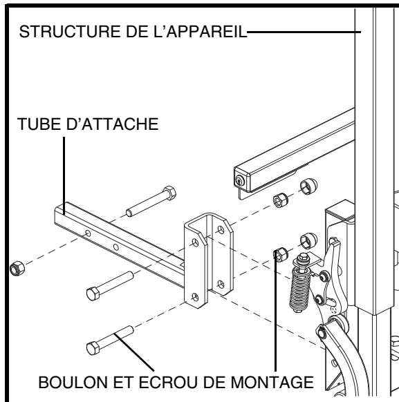
Figure 5. Ensemble du tube d'attache
