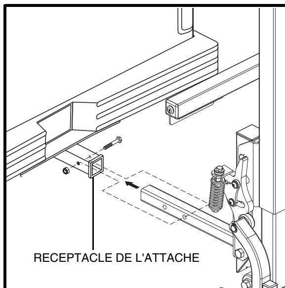
Figure 6. Installation de la structure de l'appareil de levage sur le véhicule
